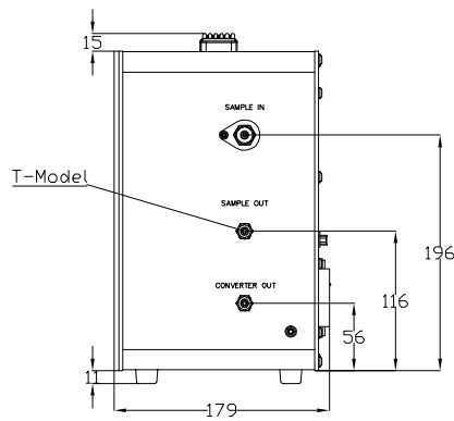
Wandmontage, Wall mount/Portabel Ansicht von Rechts Side view right
